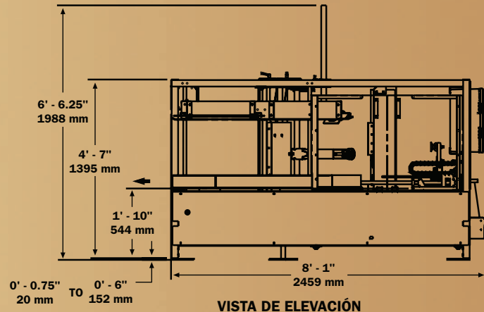
VISTA DE ELEVACIÓN
